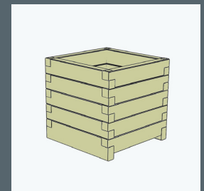
REF. BAC50 Dimensions : 50*50*50 Poids : 25 Kg
